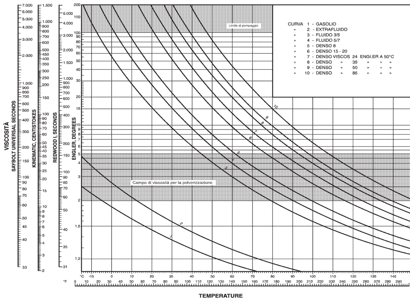
Diagramma Viscosità - Temperature
